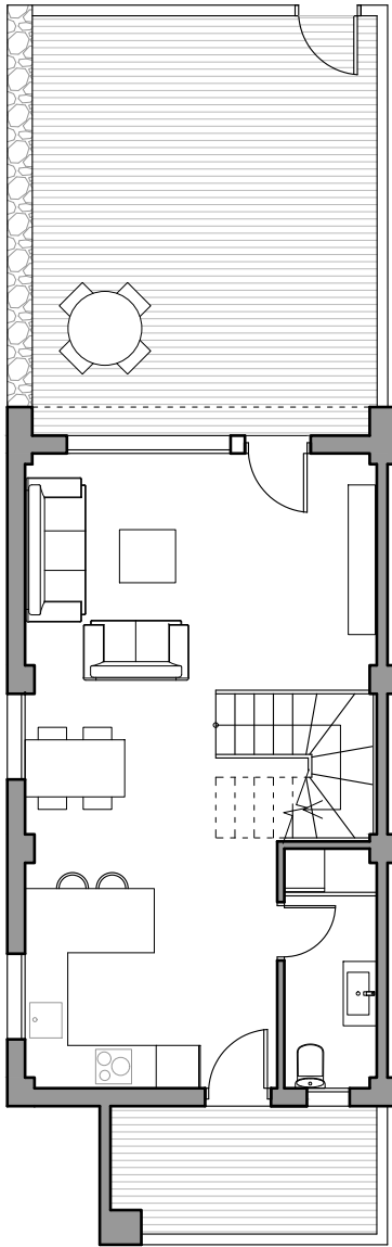
PLANTA BAJA
