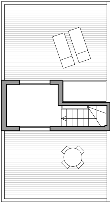
PLANTA CUBIERTA
